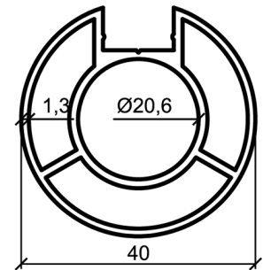
\varnothing 40 sa jednim kanalom 4,83 kg - 24.15 €
