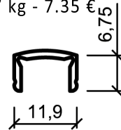
Poklopac stuba \varnothing 40 0,54 kg - 2.7 €
