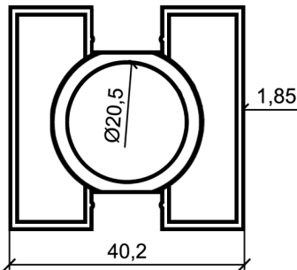
Kutijasti stub 7,38 kg - 36.9 €
