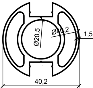
\varnothing 40 sa debljim zidom 7,38 kg - 36.9 €
