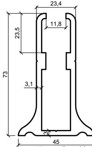
Donji nosač stakla 11,43 kg - 57.15 €
