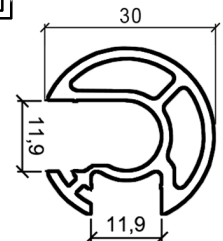
Ispuna sa 2 kanala \varnothing 30 3,8 kg - 19 €
