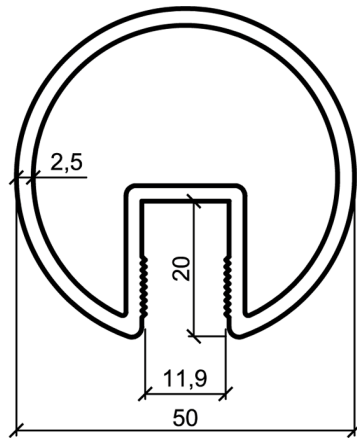
\varnothing 50 rukohvat za staklo 7,59 kg - 37.95 €
