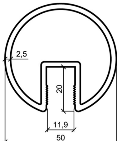
Ø50 rukohvat za staklo 7,59 kg - 37.95 €
