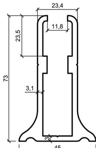
Donji nosač stakla 11,43 kg - 57.15 €
