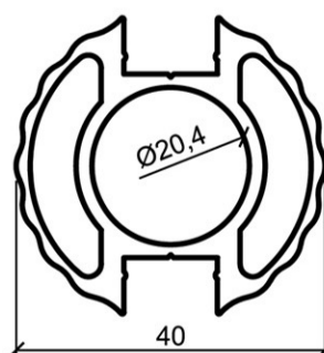
Ø40 sa ukrasnim zidom 7,38 kg - 36.9 €
