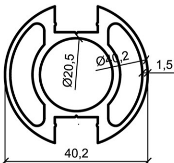
Ø40 sa debljim zidom 7,38 kg - 36.9 €
