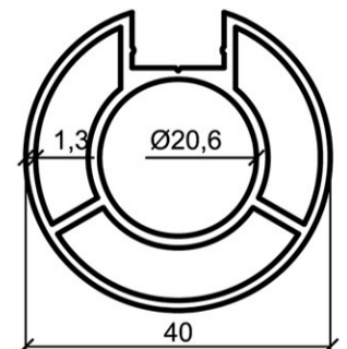
Ø40 sa jednim kanalom 4,83 kg - 24.15 €
