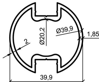
Ø40 lakši 5,1 kg - 25.5 €
