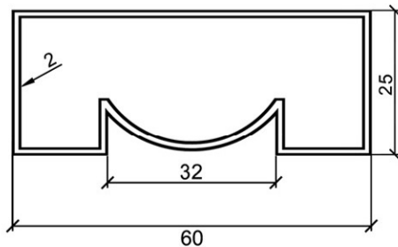
Kutijasti rukohvat 6,1 kg - 30.5 €
